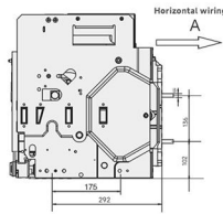
Standard horizontal wiring
